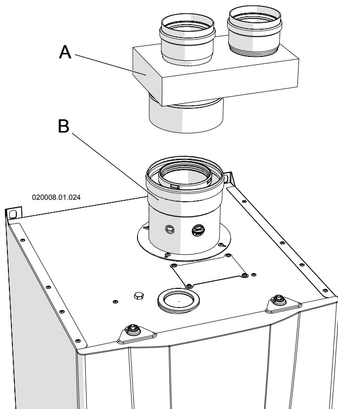
Obrázek 5-9 - Instalace systému s dvojitou trubicí „80/80PP Twin-pipe“ u modelu ICW 60
