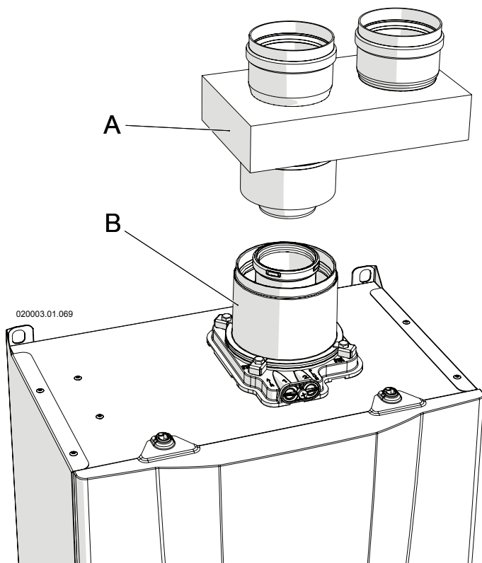
Obrázek 5-8 - Instalace systému s dvojitou trubicí „80/80PP Twin-pipe“ u modelu ICW 25 a 35
