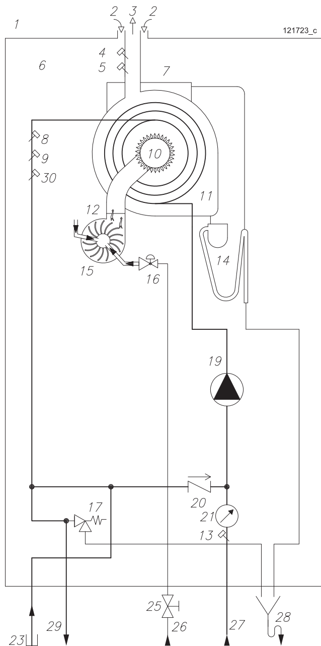
Obrázek 4-1 - Hydraulické schéma
