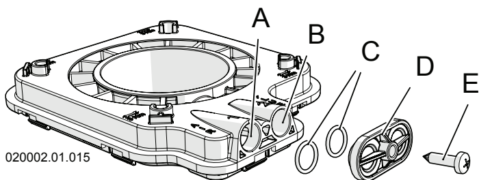
Obrázek 6-10 - Měřicí místo pro analýzu spalování u modelu ICW-25 a 35
