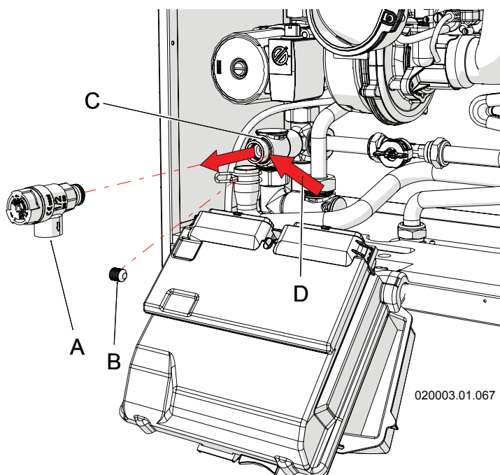
Obrázek 8-9 - Vyjmutí pojistného ventilu
