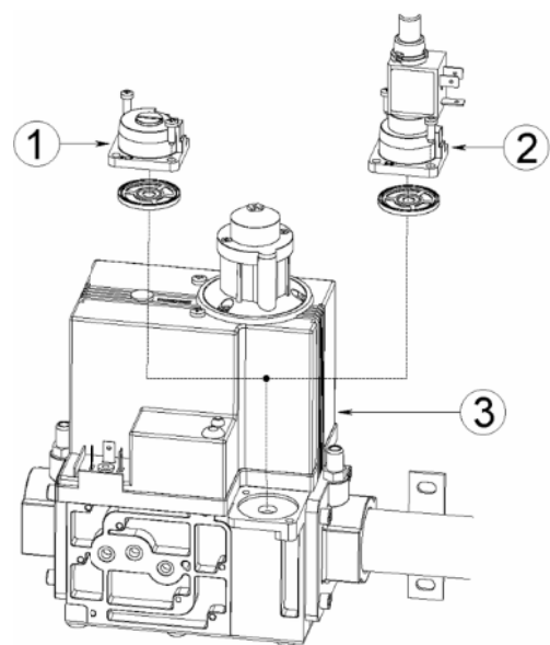
obr. 10 - prestavba plynovej armatúry
