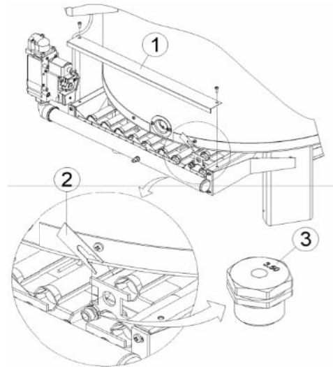
obr. 9 - výmena dýz
