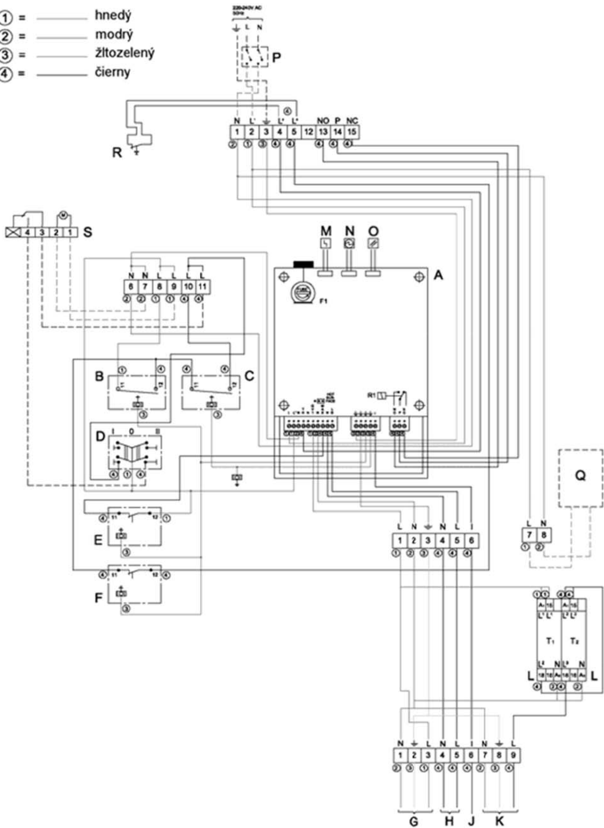
obr. 13 - schéma elektrického zapojenia Q7E-65-500 na BP
