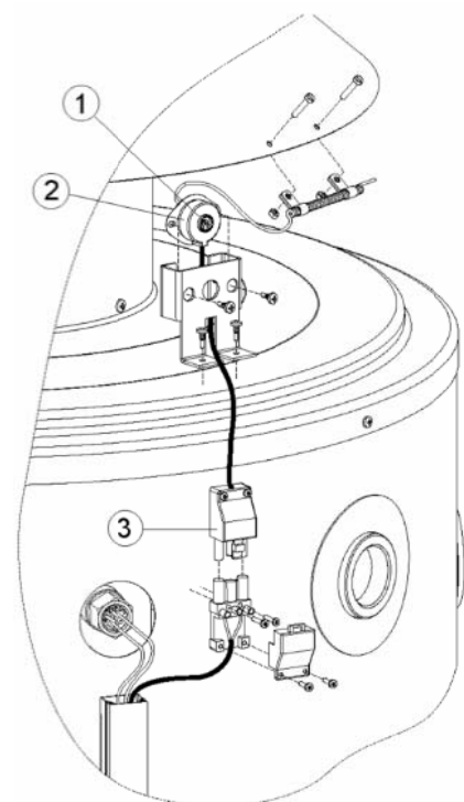
obr. 5 - montáž termostatu proti spätnému toku spalín
