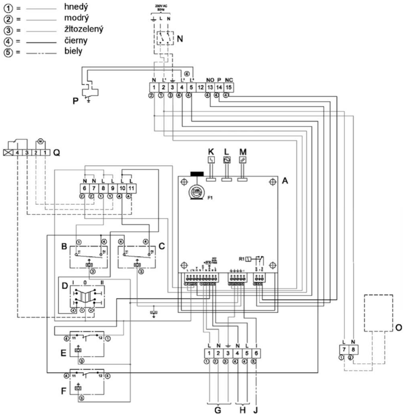
obr. 12 - schéma elektrického zapojenia Q7E-65-500 na ZP
